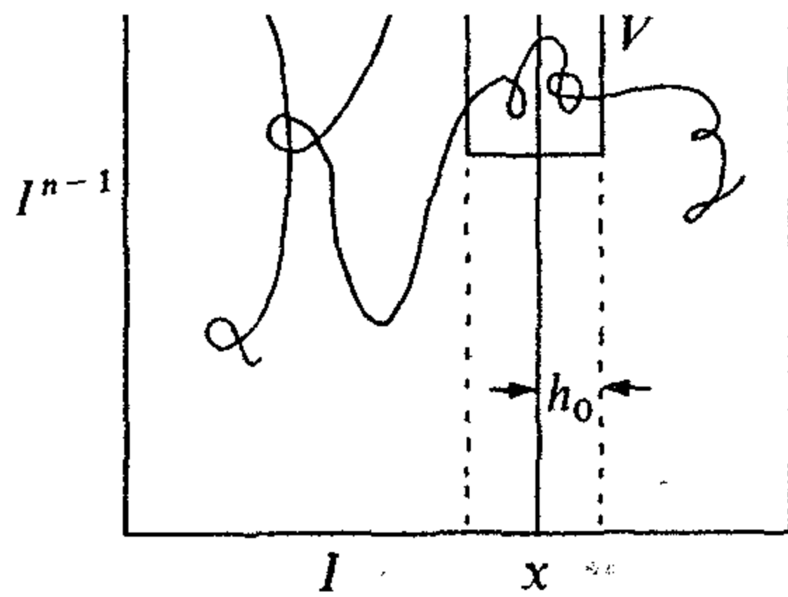
Figure C-1. Piccolo Fubini.
