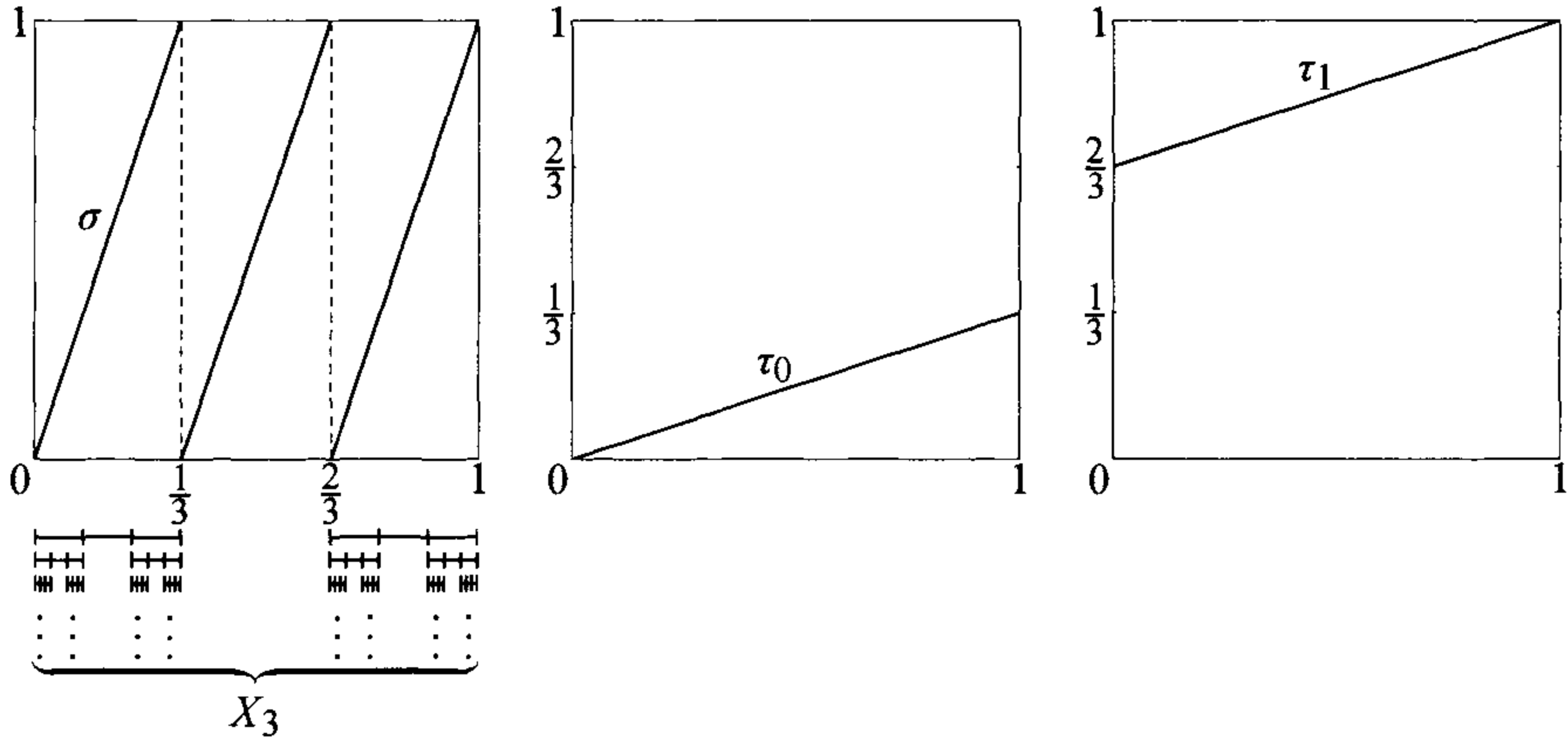
Fig. 4.2. The Cantor set X_3 .
