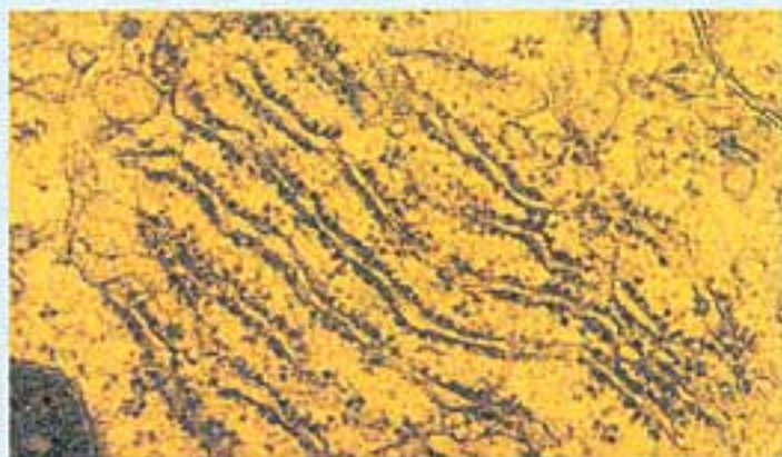
图3-5 内质网
